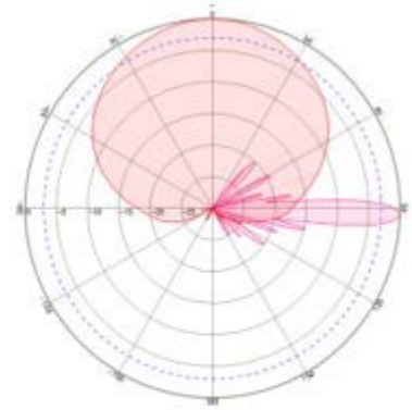
1710-2170MHz
